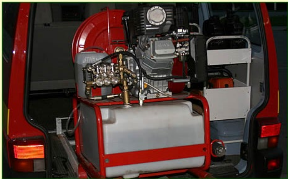
Mit dem Hochdrucklöschgerät HDL-170 können Kleinbrände, z. B. in Wohnungen und Pkws, effektiv bekämpft werden.
